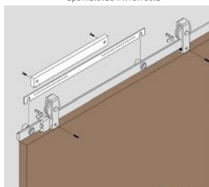
zpomalovač IN.15.900.S
